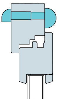
Einbau im Rahmen
