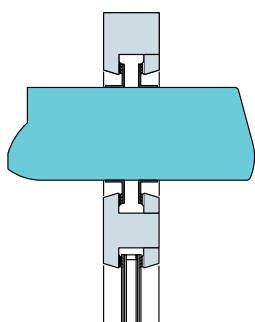
Einbau im Kämpfer
