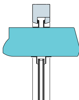
Einbau im Glasfalz
