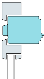
Einbau im Kämpfer
