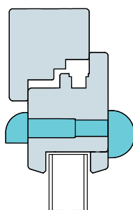
Einbau im Flügel
