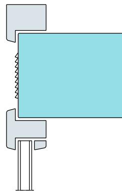
Einbau im Kämpfer
